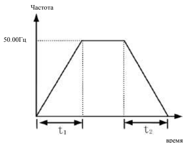
Рис. 7-1. Лinéйное ускорение и замедление
