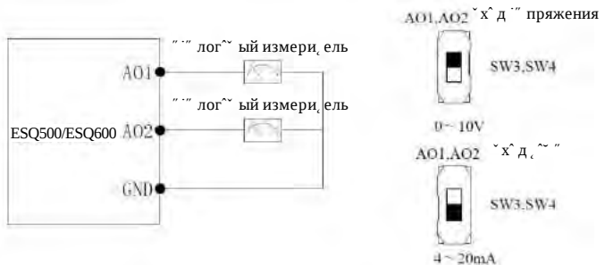
Рис.3-13 Схема монтажа клемм AO1,AO2
