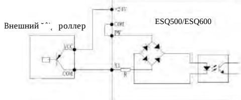
Рис. 3-15 Режим подключения со стоком на 24В 2. Для изоляции внешнего источника питания 5~30В от преобразователя и режим подключения внешнего инвертера типа NPN-типа (уберите короткую перемычку между клеммами PW и +24V).
