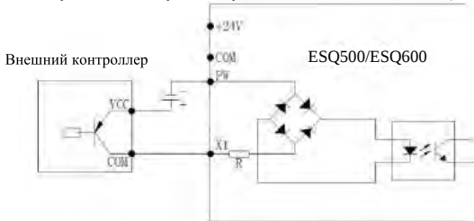
Рис.3-17 Режим подключения с внешним источником питания типа сток
