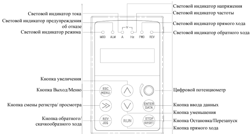
Рис.С-8 Схема пульта управления EN-LED3-D
