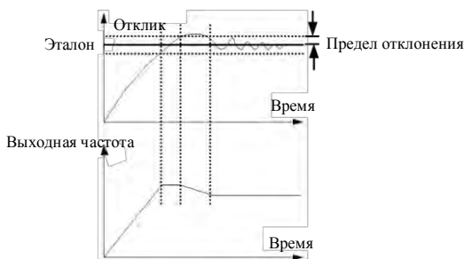
Рис.7-39 Предел отклонения
