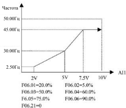
Рис. 7-11 AI1 выбирает установку частоты кривой 1
