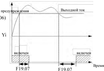
Рис.7-45 Сигнализация перегрузки
