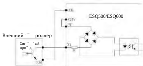
Рис.3-14 Режим подключения со встроенным источником питания на 24В 2. Для изоляции преобразователя от источника питания +24В режим подключения внешнего инвертера типа PNP-типа.
