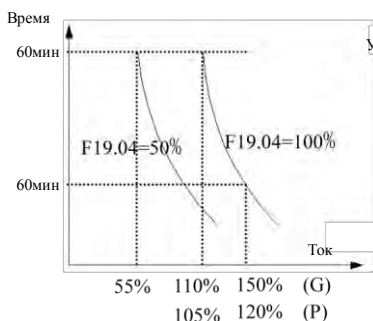
Рис.7-44 Защита электронным тепловым реле
