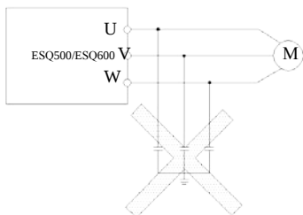
Рис.1-2 Запрещено устанавливать конденсатор на выходной стороне
