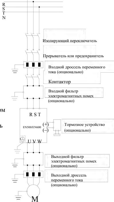
Рис.3-8 Соединение преобразователя и сопрягаемых деталей
