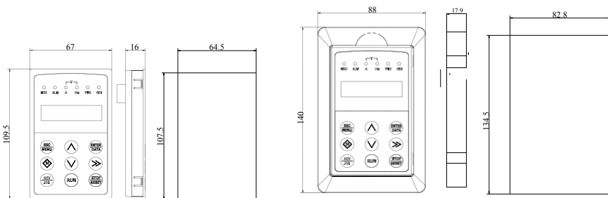
Рис.2-7 Монтажные размеры пульта управления
