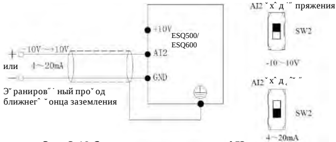
Рис. 3-12 Схема монтажа клеммы AI2
