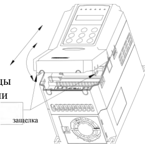
Рис.3-4 Демонтаж и сборка металлической крышки
