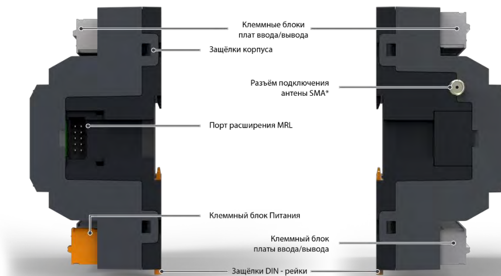
Рис. 3 – Контроллер Matrix. Виды сбоку
