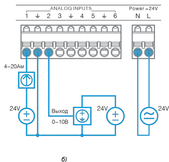
Рис. 18 - Подключение активных датчиков с питанием от одного источника (а); от отдельных источников (б)
