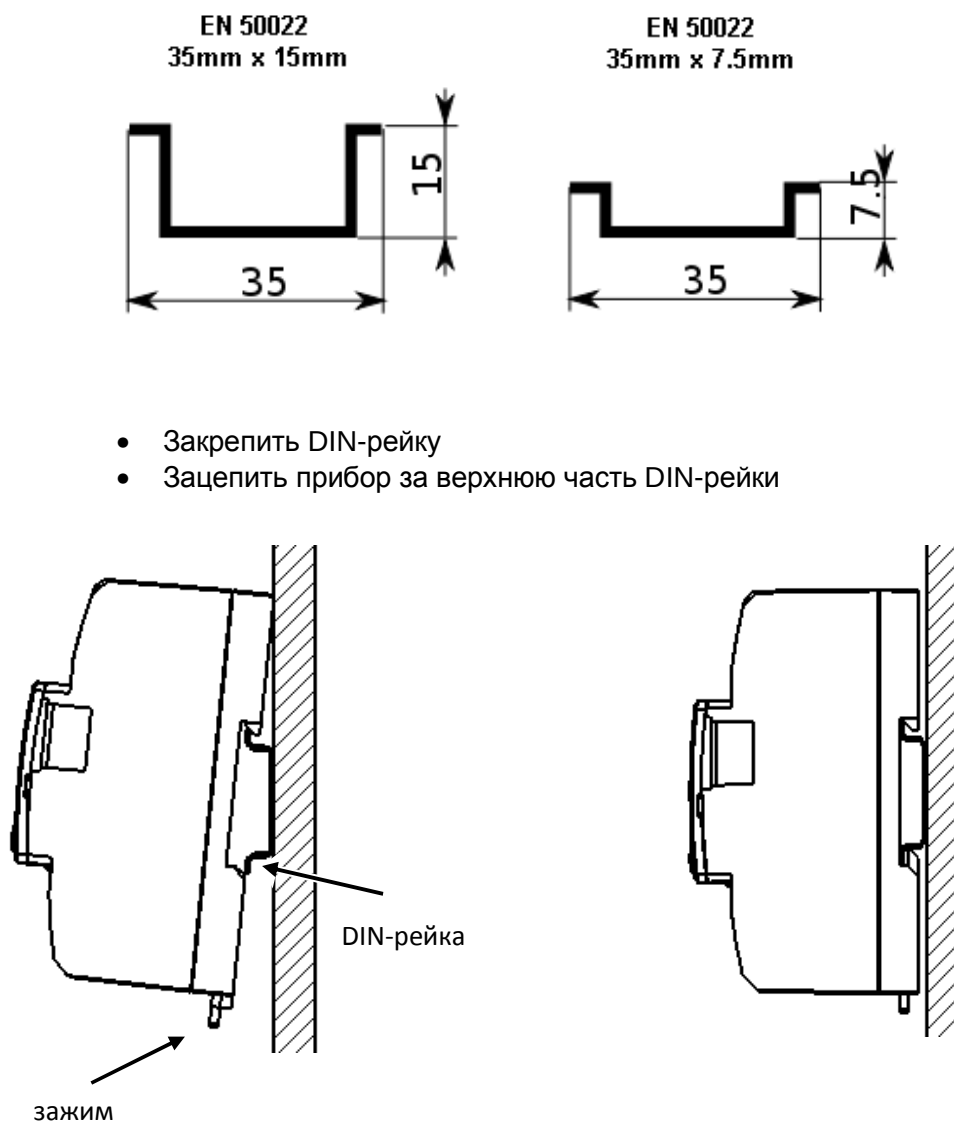
Рисунок 14. Установка контроллера на рейку
