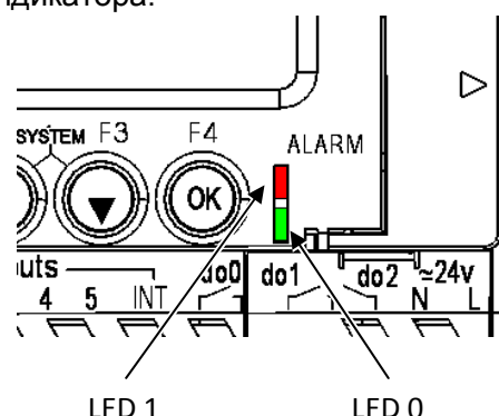
Рисунок 3. Внешняя светодиодная индикация
