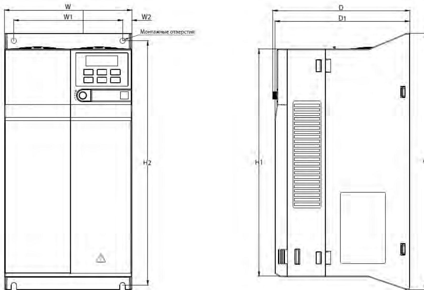
Рис.2-6.4. Чертеж преобразователя частоты типоразмер А4
