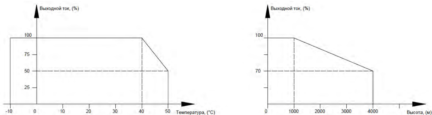
Рис. 2-4. Снижение характеристики преобразователя частоты при превышении допустимой температуры и высоты
