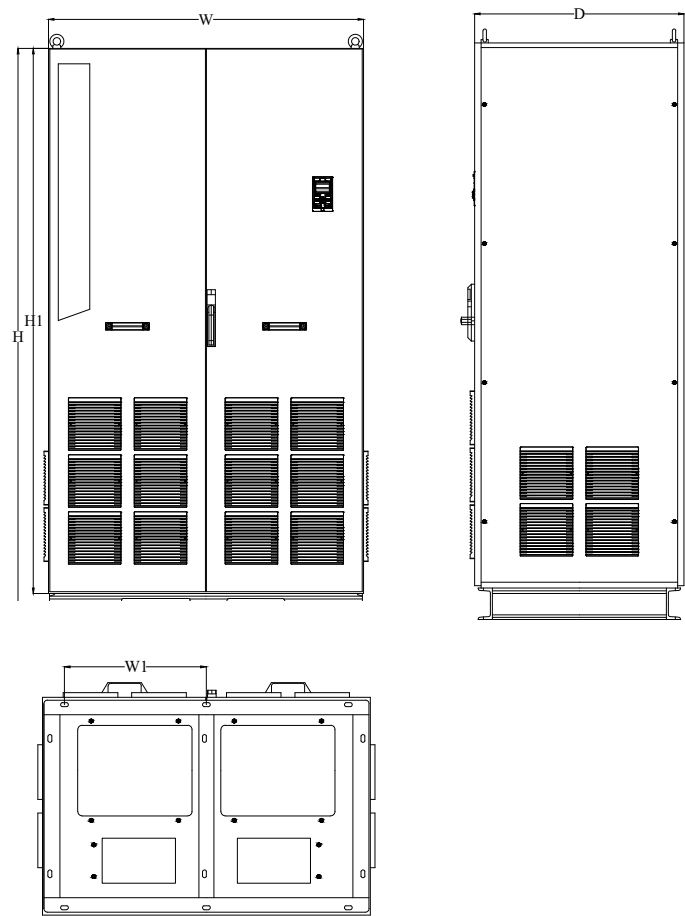
Типоразмер В13 (630 – 1120 кВт) НО - высокая перегрузка, NO - нормальная перегрузка
